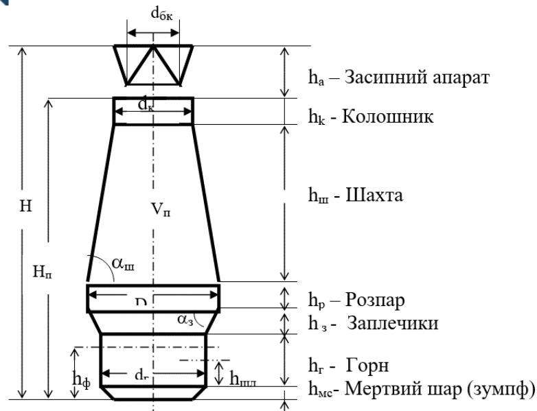
Рисунок 1.3 – Схема профілю доменної печі і його розміри:
