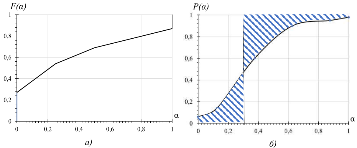
Рисунок 2 – Функція розподілу зростків в початковому матеріалі (а) та сепараційна характеристика процесу розділення (б)
