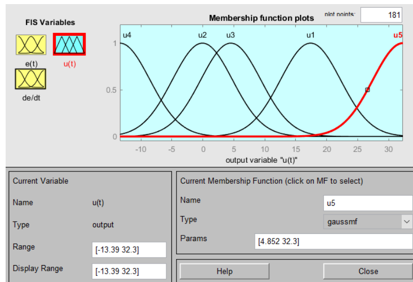
Рисунок 2.12 – Результат налаштування функцій приналежності вихідної змінної
