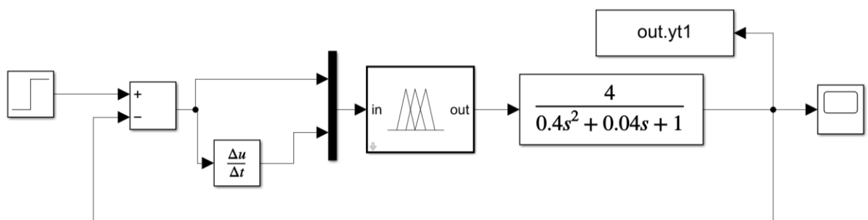
Рисунок 2.16 – Математична модель синтезованої нечіткої системи управління
