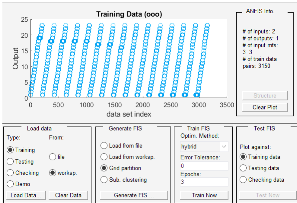
Рисунок 1.4 - Результат завантаження бази даних до модуля ANFIS
