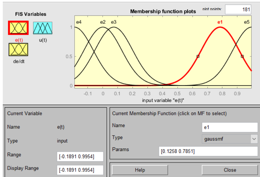
Рисунок 2.10 – Результат налаштування функцій приналежності вхідних змінних «Помилка управління»
