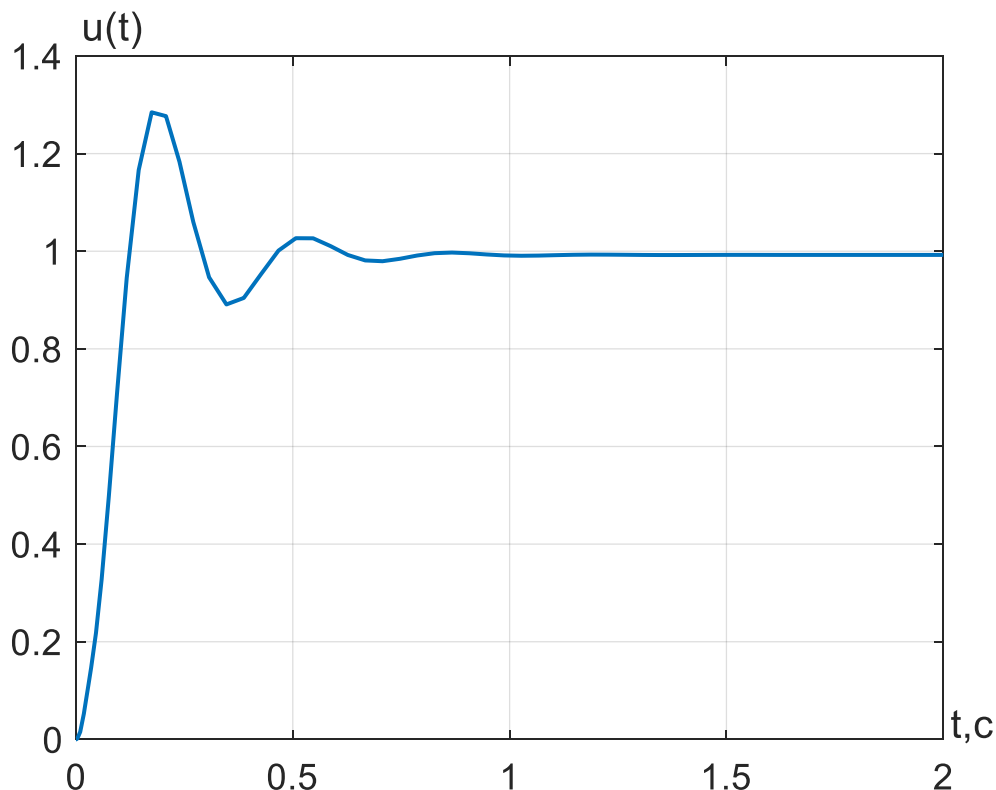
Рисунок 2.28 – Перехідний процес під управлінням синтезованого НЛР
