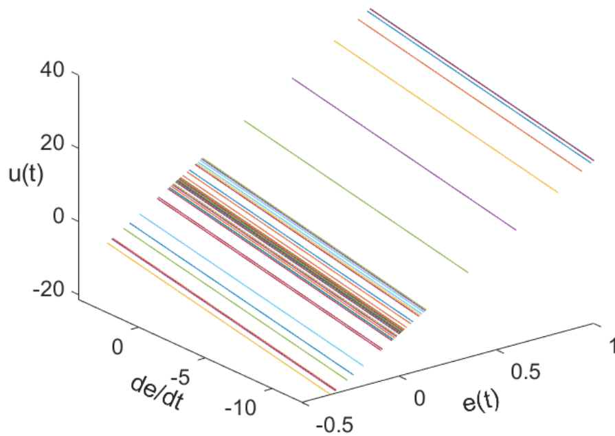
Рисунок 2.8 – Поверхня відгуку ПД-регулятора
