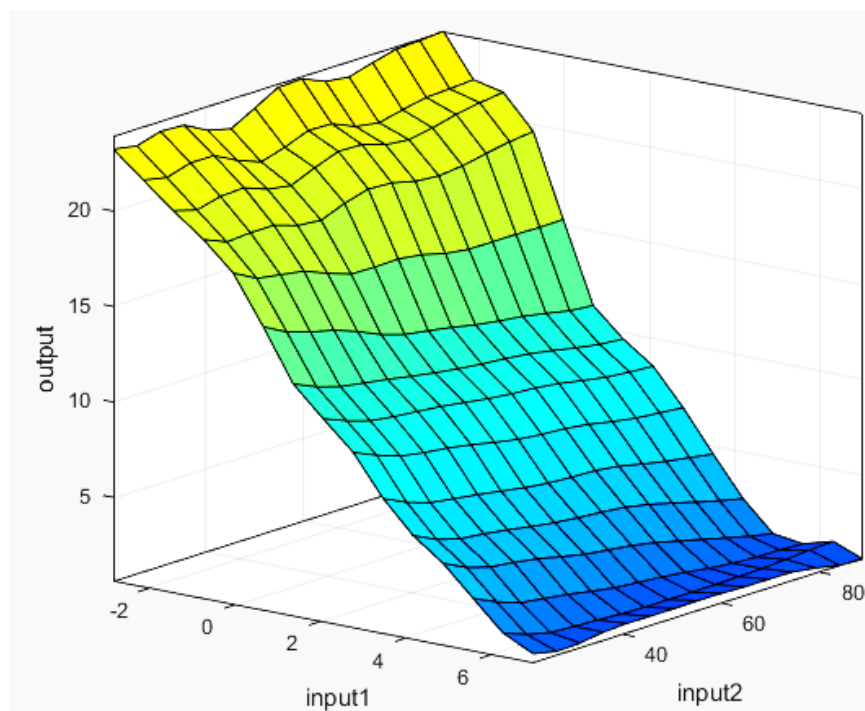
Рисунок 1.13 - Графічне подання закону управління
