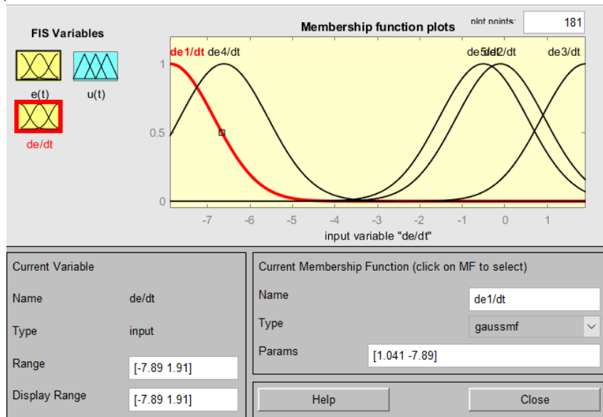
Рисунок 2.11 – Результат налаштування функцій приналежності вхідних змінних «Похідна помилки управління»
