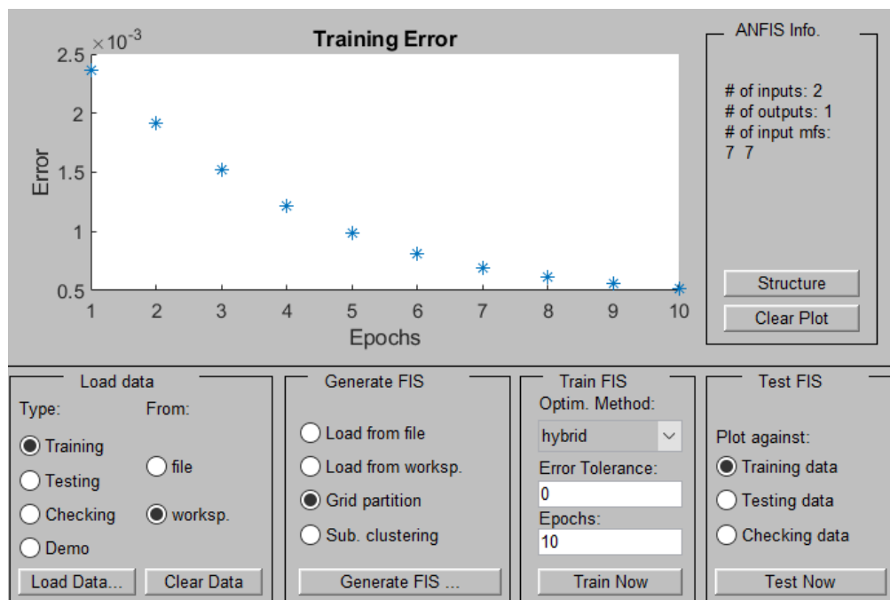
Рисунок 2.21 - Проміжні результати навчання
