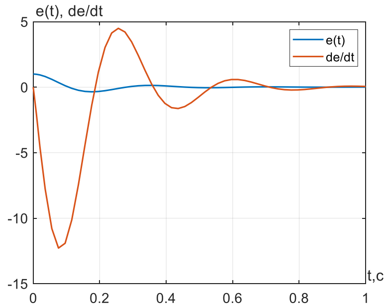
Рисунок 2.6 – Графік зміни помилки та її похідної
