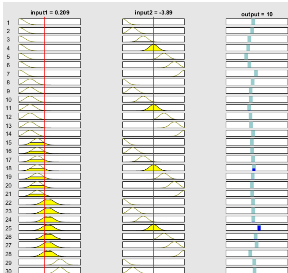
Рисунок 2.26 - Робота системи нечіткого висновку
