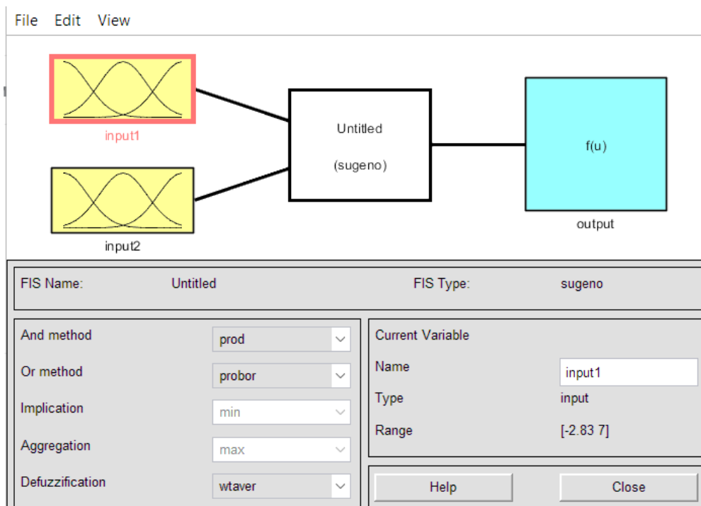
Рисунок 1.9 – Згенерований інтерфейс FIS editor
