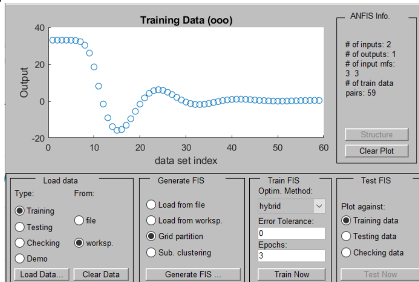
Рисунок 2.18 - Результат завантаження бази даних до модуля ANFIS
