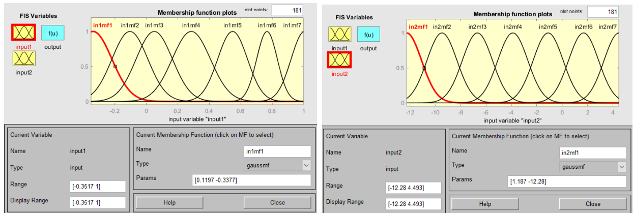
Рисунок 2.24 – Результат налаштування функцій приналежності вхідних змінних
