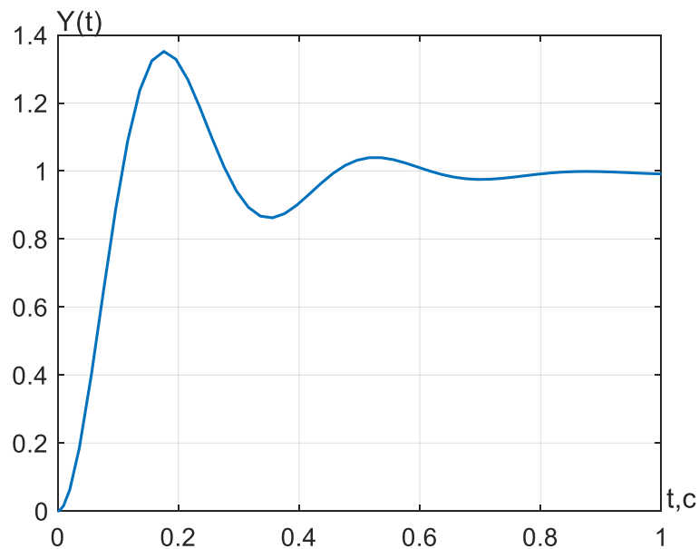
Рисунок 2.5 – Графік перехідного процесу системи управління з ПД-регулятором
