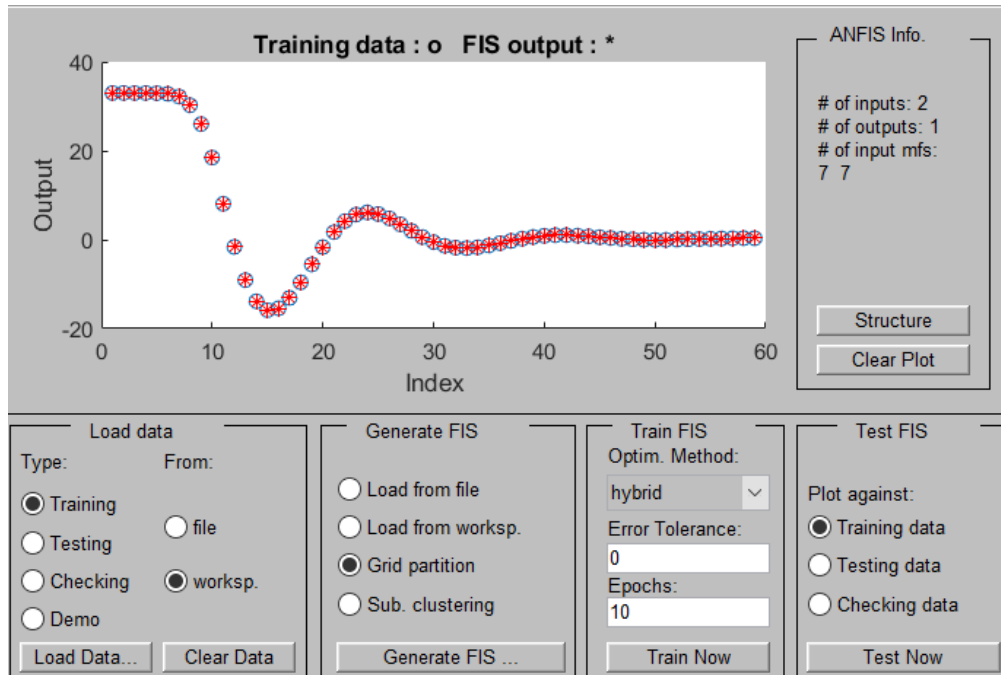
Рисунок 2.22 – Результати тестування нечіткої системи
