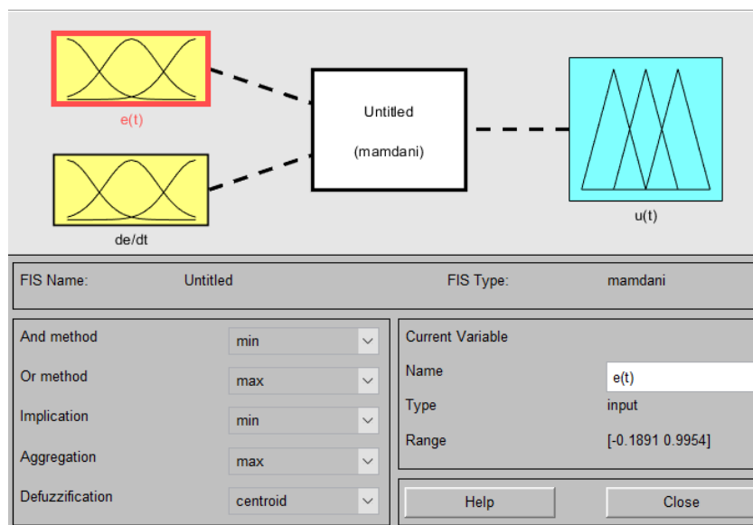
Рисунок 2.9 – Налаштуємо редактор системи нечіткого висновку FIS editor
