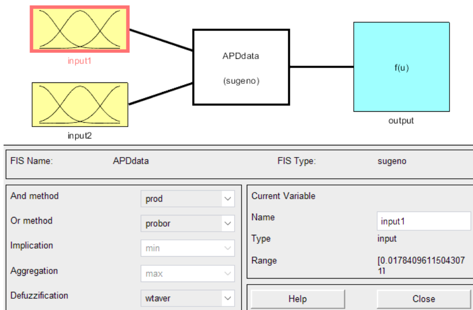
Рисунок 2.23 – Згенерований інтерфейс FIS editor
