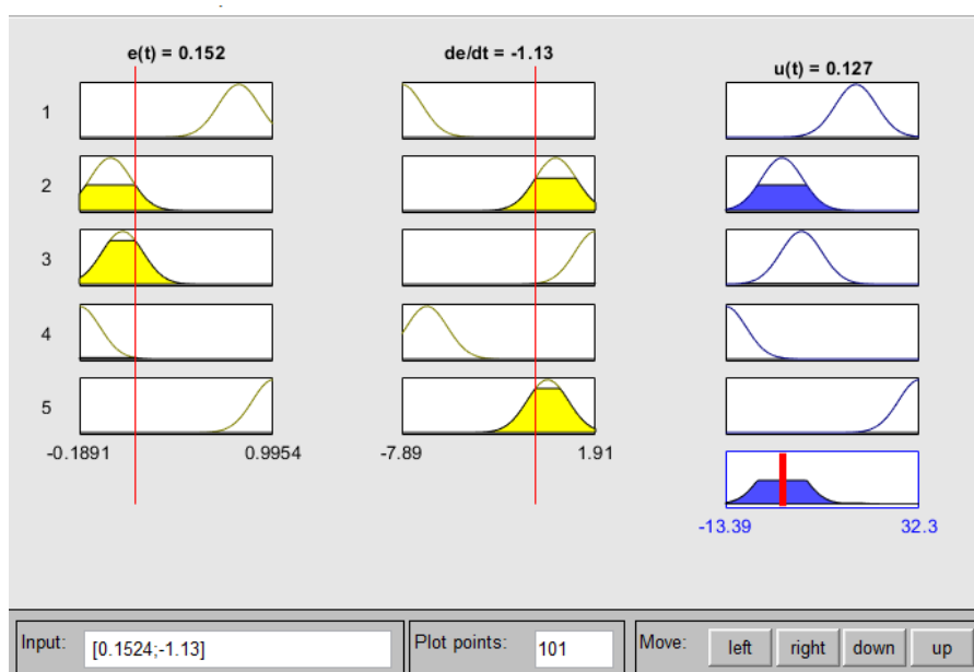
Рисунок 2.14 - Робота системи нечіткого супервізора НЛР_ПД
