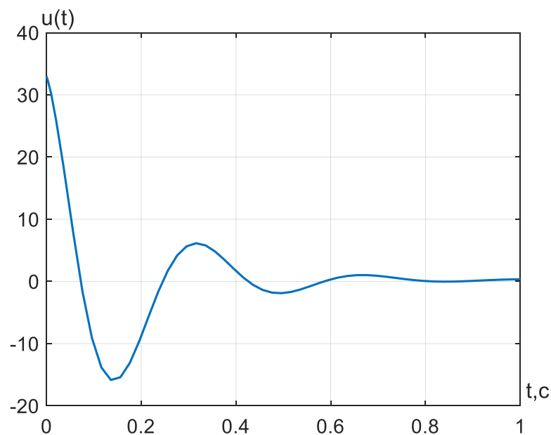
Рисунок 2.7 – Графік зміни сигналу управління за час перехідного процесу
