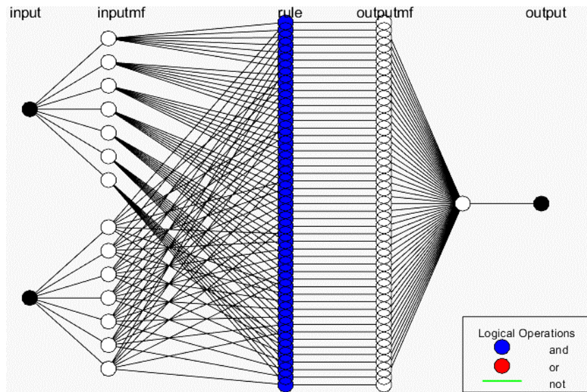
Рисунок 2.20 – Згенерована нейронечітка структура
