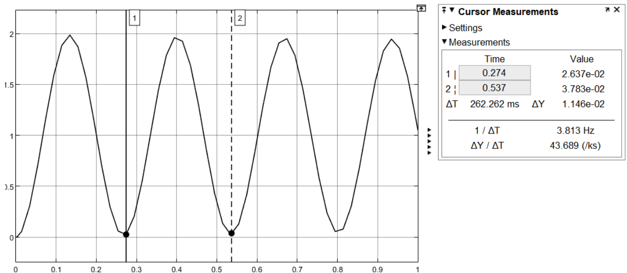
Рисунок 2.3 - Графіку перехідного процесу при налаштуванні ПД-регулятора методом Зиглера-Нікольса ( K_D=0 , K_P=55 )
