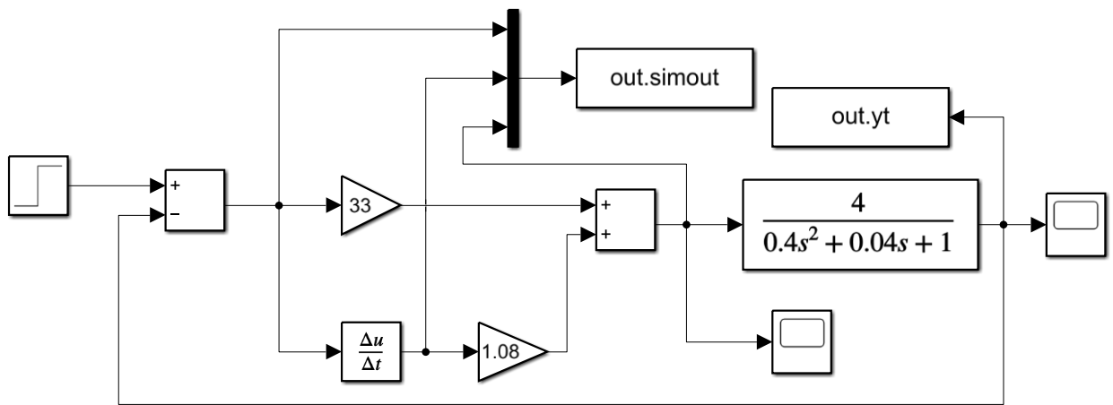
Рисунок 2.4 – Математична модель системи управління з ПД-регулятором
