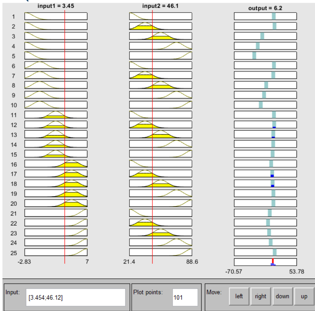
Рисунок 1.12 - Робота системи нечіткого висновку
