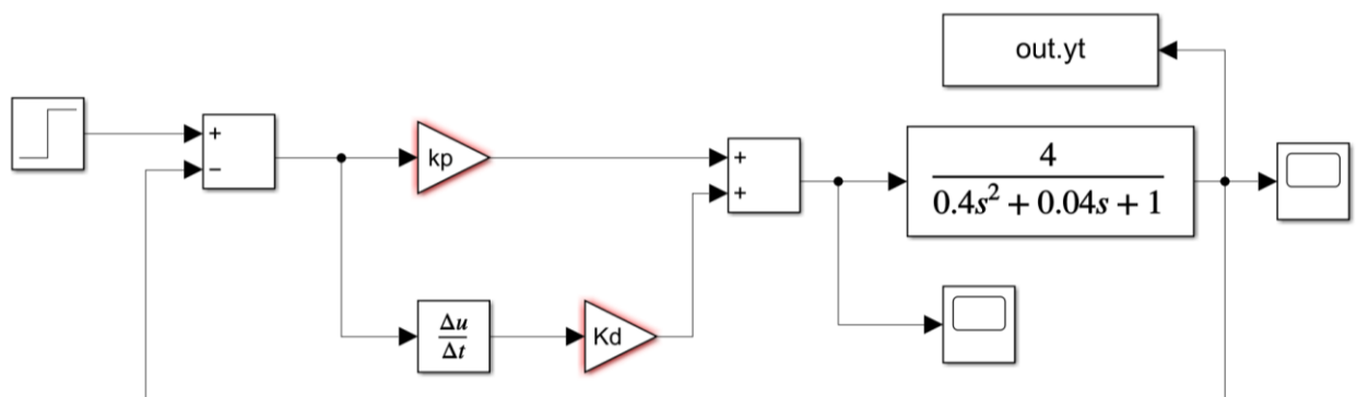
Рисунок 2.1 – Структурна схема системи управління з ПД-регулятором
