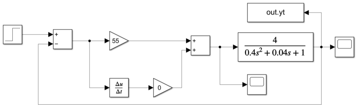
Рисунок 2.2 – Налаштування коефіцієнтів передачі ПД-регулятора методом Зиглера-Нікольса
