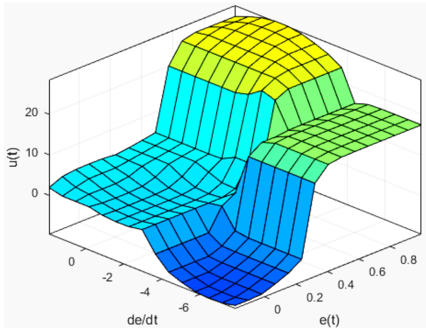
Рисунок 2.15 - Графічне подання закону управління
