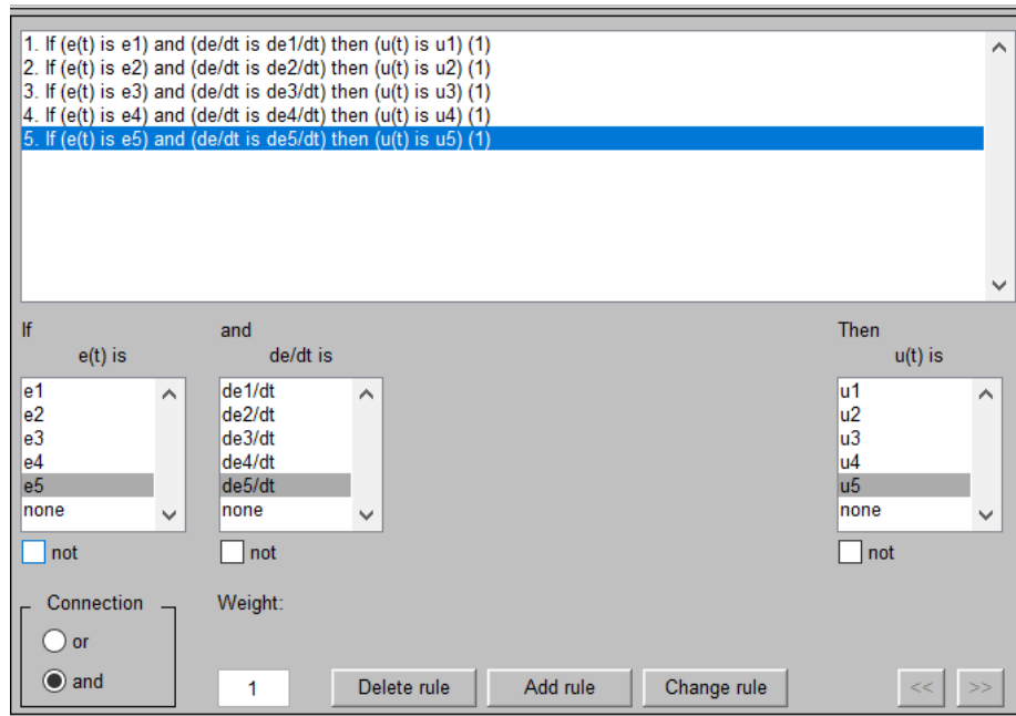
Рисунок 2.13 - Налаштовування опису правил функціонування нечіткого НЛР_ПД за експериментальними даними
