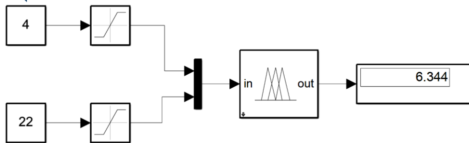
Рисунок 1.14 - Simulink модель функціонування згенерованої нечіткої системи управління за базою даних
