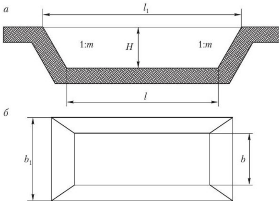
Рисунок 2.3 – Розрахункова схема кар'єру: а – поздовжній розріз кар'єру; б – план; b , b_1 - ширина; l , l_1 – довжина; розміри поверху; H – глибина кар'єру
