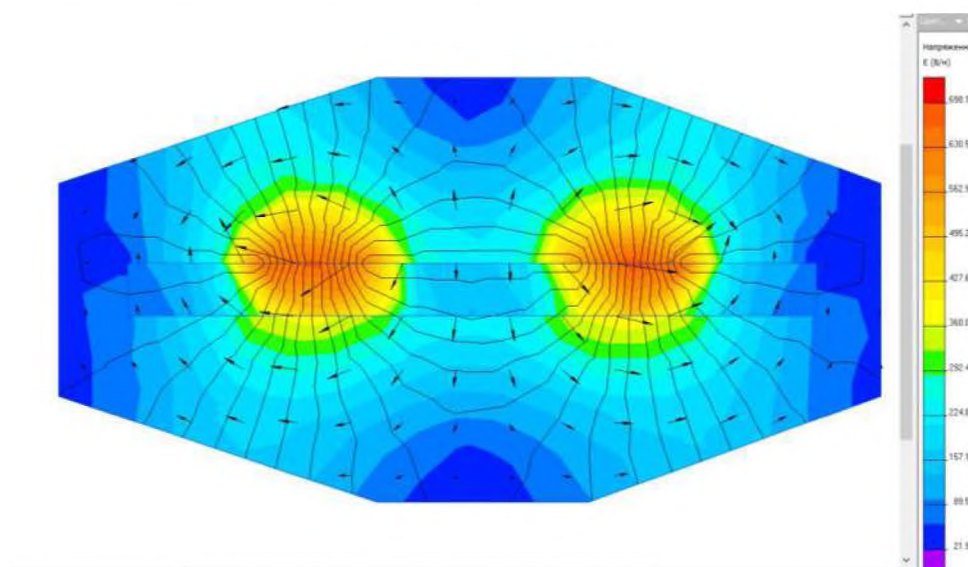
Рис. 2. Картина розподілу електростатичного поля при сухому ґрунті ( \epsilon = 2 )
