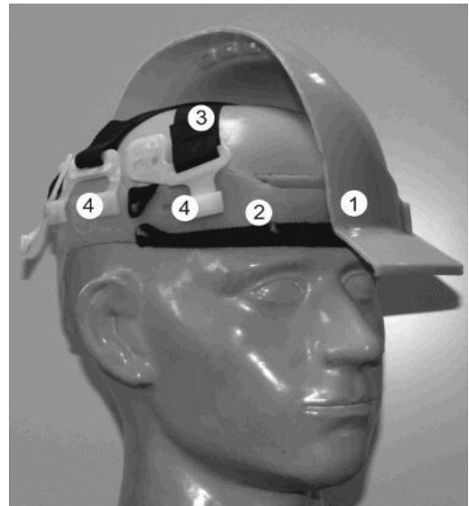
Рисунок 7.3 – Конструкція промислового захисної каски: 1 – захисний корпус, 2 – амортизатор, 3 – фіксатори амортизатора, 4 – наголів'я, 5 – вентиляційні отвори, 6 - козирок, 7 – фіксуєчий ремінь.
