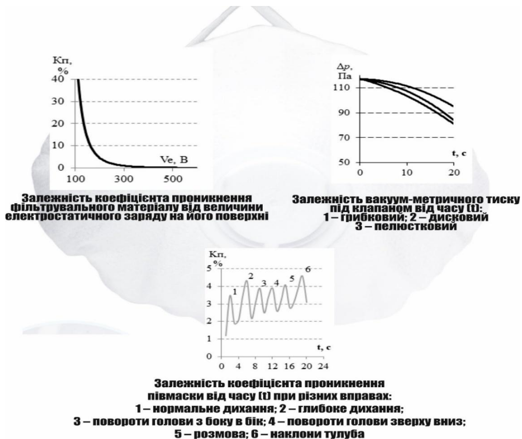
Рисунок 4.7 – Лабораторні дослідження показників конструктивних елементів та готових фільтрувальних півмасок[26]
