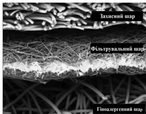
Рисунок 2.8 – Конструкція фільтрів респіратора: зовнішній захисний шар (1); попередній фільтр (2); основний фільтр (3); гіпоалергенний шар (4)
