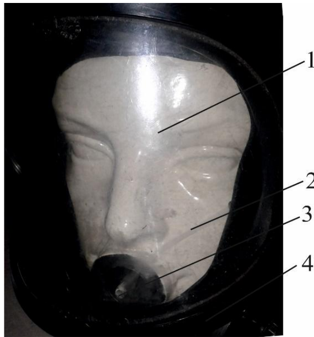
Рисунок 2.1 – Вигляд цівки аерозолю, що проникає крізь обтюратор: 1 – маска; 2 – цівка аерозолю; 3 – повітрязабірник; 4 – обтюратор
