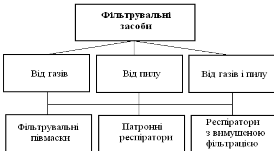
Рисунок 3.7 – Класифікація ЗІЗОД за принципом дії і призначенням відповідно до НПАОП 0.00-1.04-07[22]
