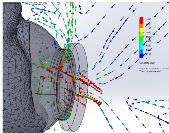
Рисунок 4.12 – Приклад моделювання потрапляння запылених потоків до півмаскового простору[37]
