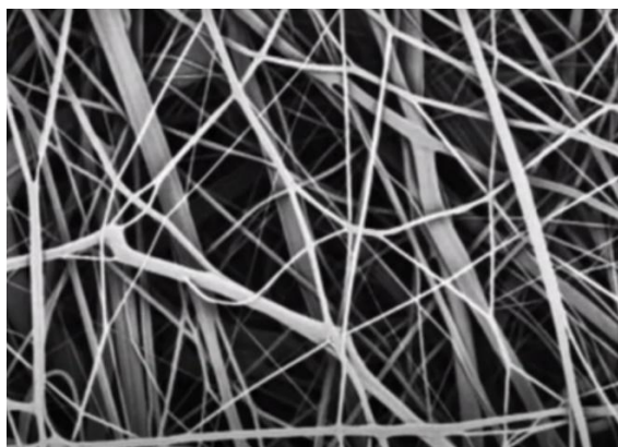
Рисунок 2.9 – Структура фільтрувального матеріалу (збільшення в 300 разів)
