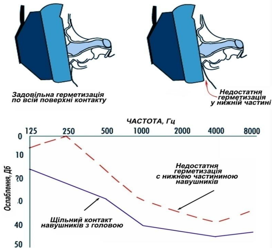
Рисунок 9.3 – Правильне і неправильне положення навушників і відповідне ослаблення рівня шуму[40,42]
