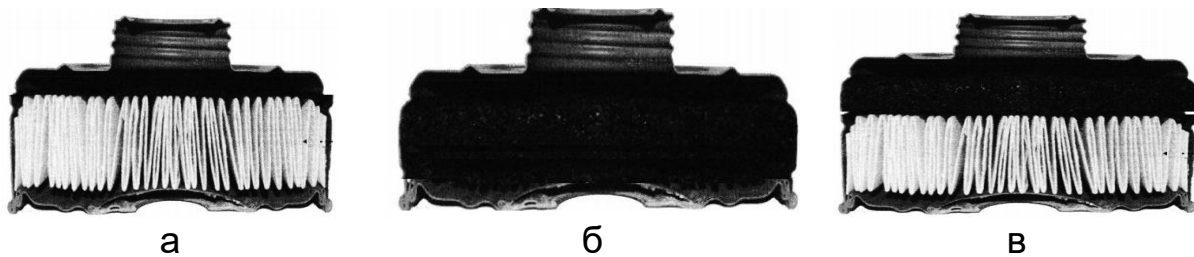
Рисунок 3.2 – Фільтрувальні елементи до ЗІЗОД протипилові (а), протигазові (б); комбіновані (в)
