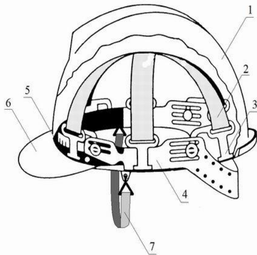
Рисунок 7.3 – Конструкція промислового захисної каски: 1 – захисний корпус, 2 – амортизатор, 3 – фіксатори амортизатора, 4 – наголів'я, 5 – вентиляційні отвори, 6 - козирок, 7 – фіксуєчий ремінь.
