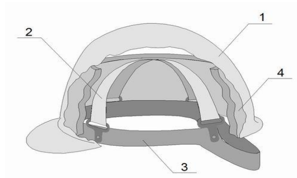
Рисунок 7.5 – Конструкція високоякісного захисного шолома: 1 – захисний корпус, 2 - амортизатор, 3 – наголів'я, 4 – підсилююча захисна прокладка
