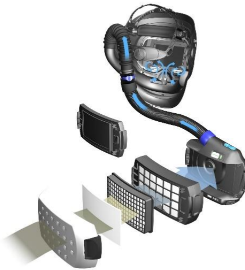
Рисунок 3.3 – Фільтрувальний ЗІЗОД з примусовою подачею повітря
