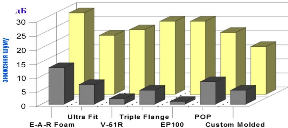
Рисунок 9.2 – Порівняння коефіцієнтів ослаблення шуму, виміряних в лабораторних умовах (далекій ряд) і на практиці (ближній ряд) у противозумних вкладишів 7 різних конструкцій [40,41]
