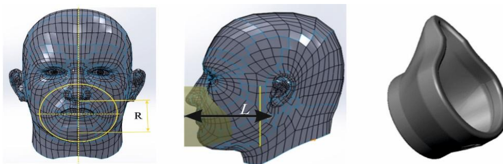
Рисунок 4.11 – Етапи побудови «NURBS»- моделі півмаски респірація[37]
