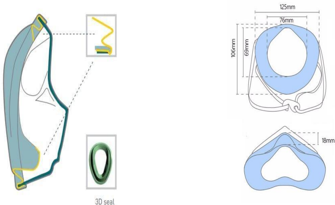
Рисунок 3.6 – Конструкції обтюраторів респіраторів зі самовисмоктування
