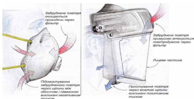
Рисунок 3.5 – Різниця між респіраторами з примусовою подачею повітря і самовисмоктуванням
