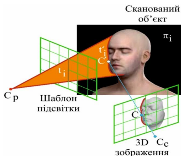
Рисунок 4.9 – Схема побудови моделі оптичної триангуляції: C_p і C_c - оптичні центри проектора і камери[37]
