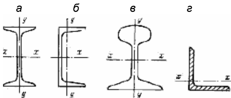
Рисунок 2.1 – Профілі прокату, які застосовують для виготовлення металевого кріплення: а) двотаврові балки; б) швелери; в) рейки; г) куткова сталь
