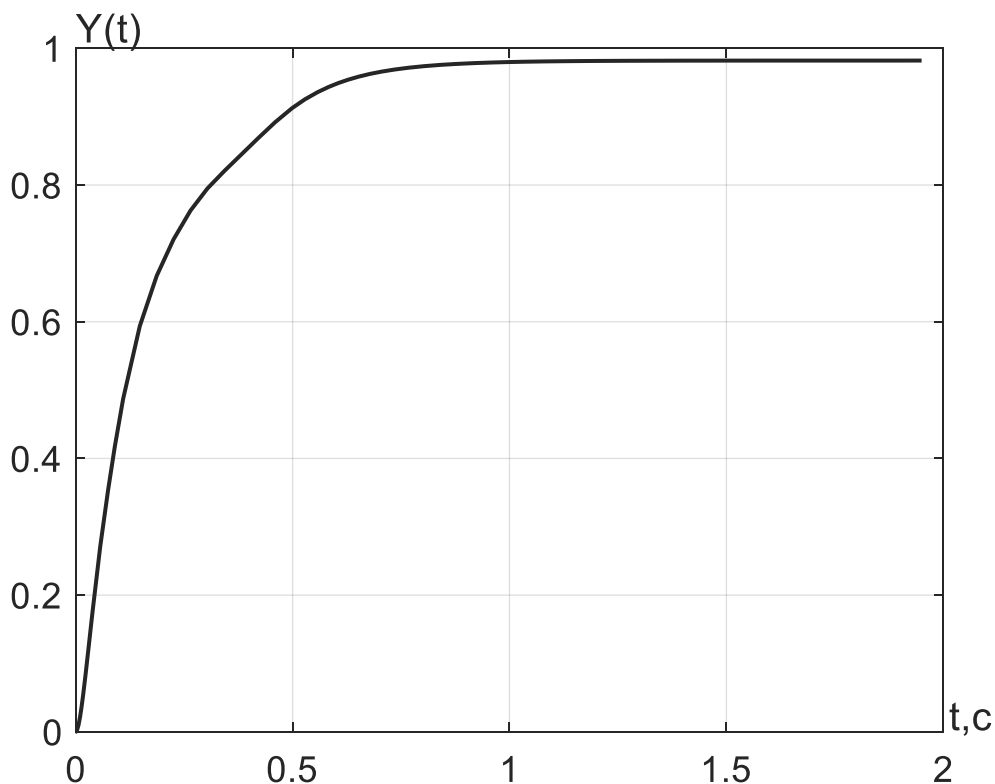
Рисунок 3.2 – Графік перехідної характеристики
