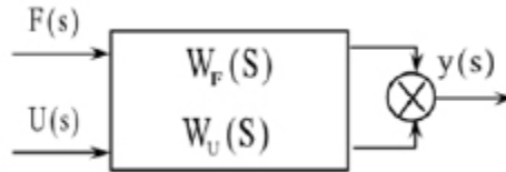
Рис. 3. Мехатронна схема керування зі зворотнім зв'язком
