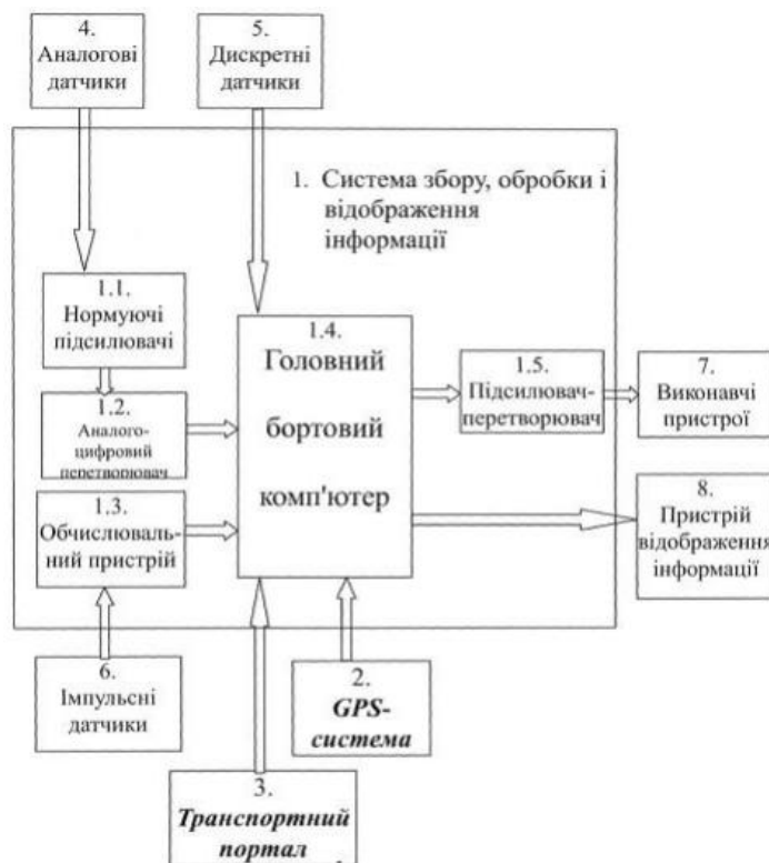
Рис. 1. Структура мехатронної системи керування
