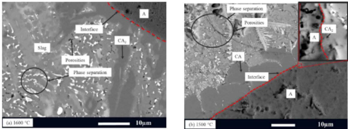
Рис. 2. Продукти реакції, що утворилися на межі поділу фаз частинки \text{Al}_2\text{O}_3 -шлак (а) при 1600\text{ }^\circ\text{C} (б) при 1500\text{ }^\circ\text{C} . Границя поділу фаз показана червоною лінією
