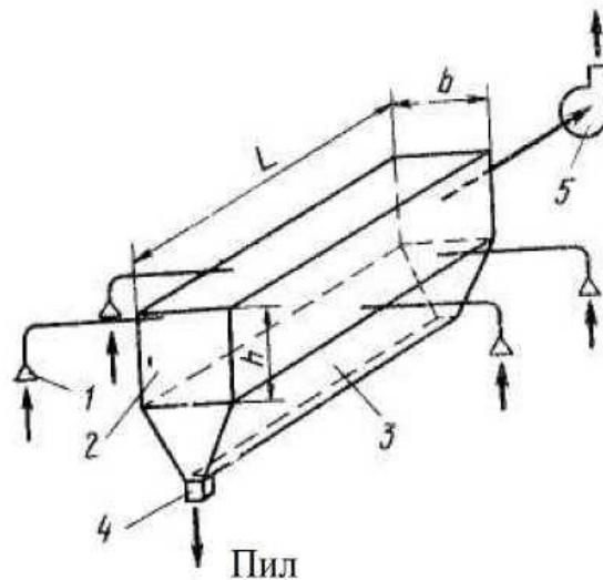
Рисунок 2.1 – Схема горизонтального колектору: 1 - відсмоктування; 2 - колектор; 3 - бункер колектору; 4 - патрубок для видалення пилу; 5 - вентилятор
