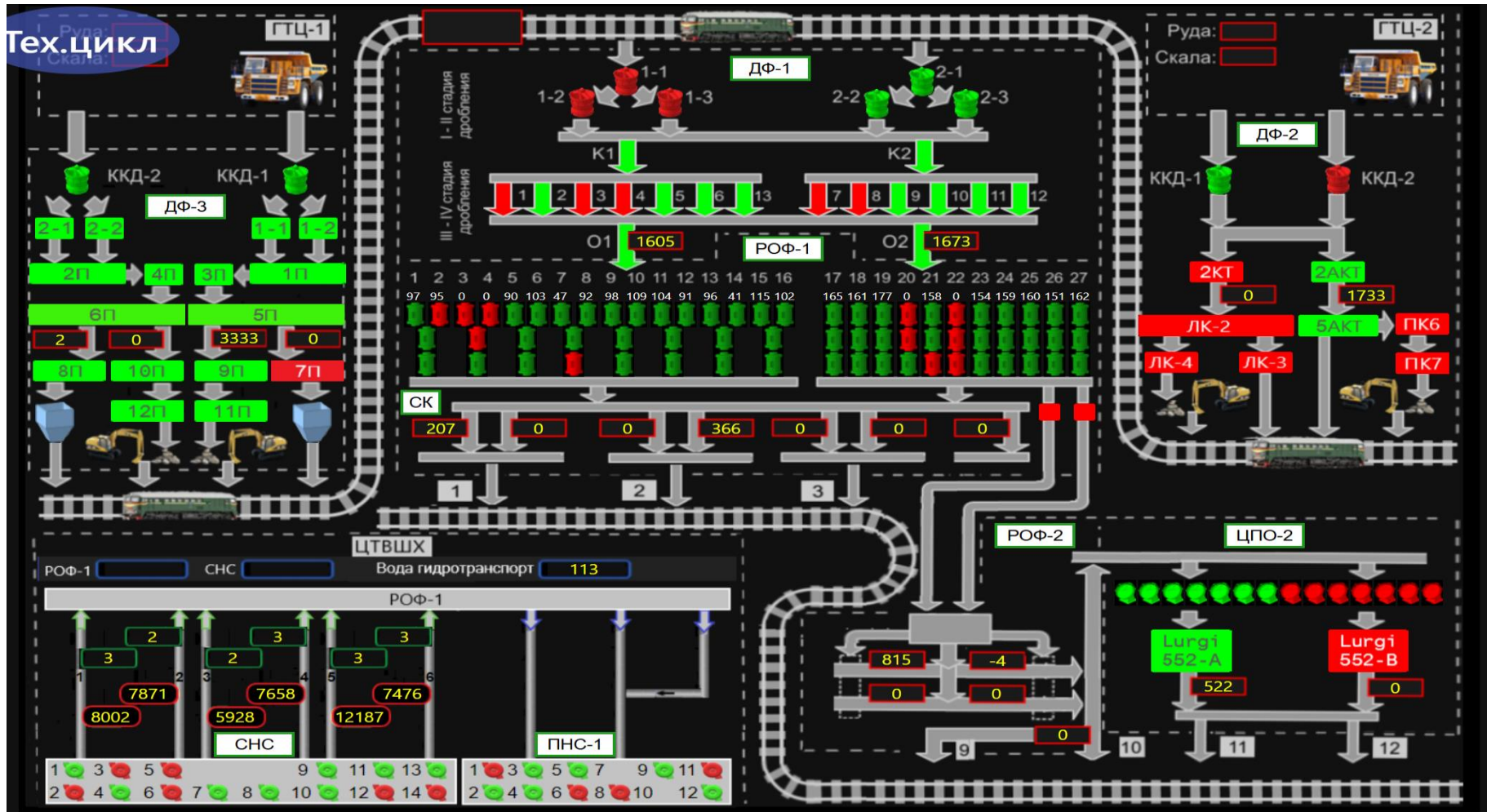
Рисунок 1.1 – Технологічний цикл переробки магнетитових кварцитів на «Північному ГЗК»
