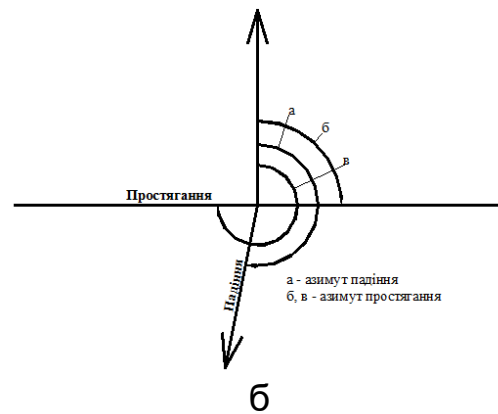
Рисунок 4.1 – Елементи залягання шарів гірських порід у відслоненні (а) і на плані (б).
